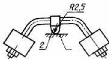
1 - образец; 2 - сферическая часть
