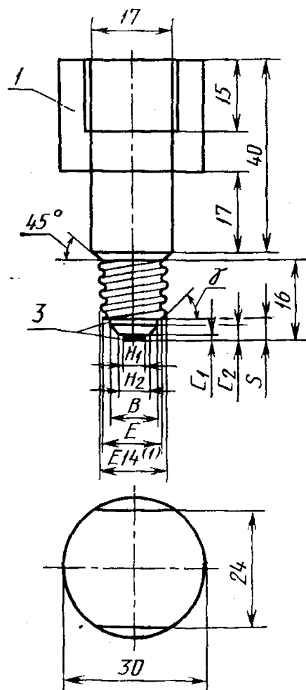
Испытательный цоколь А
