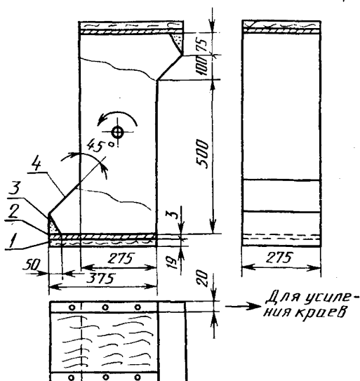
1 — беревая плита; 2 — сталь; 3 — резина; 4 — гладкий пластмассовый лист
