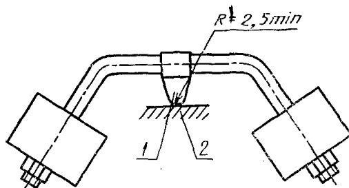
1 — сфера; 2 — образец
