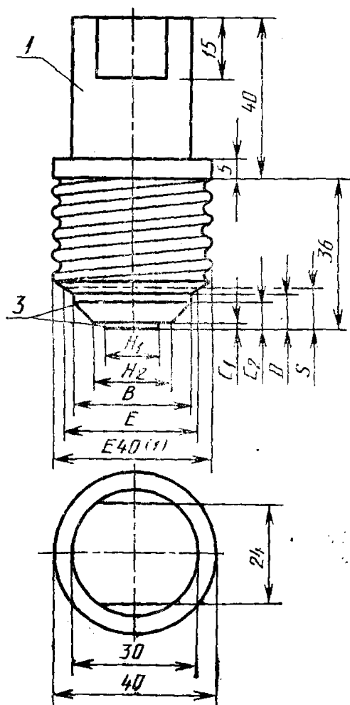
Испытательный цоколь А
