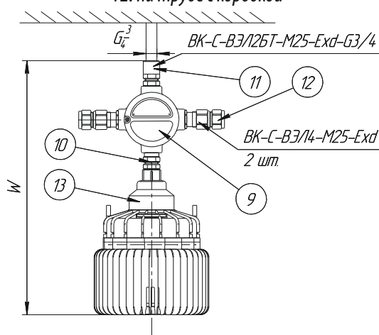
T2: на трубе с коробкой
