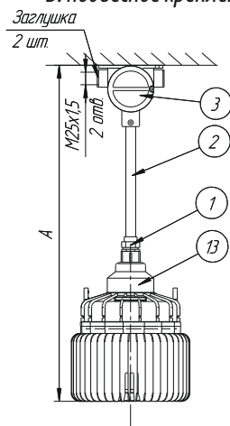
В: подвесное крепление
