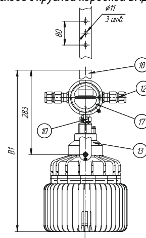
C2: на скобе с круглой коробкой ВАД-РСП-С
