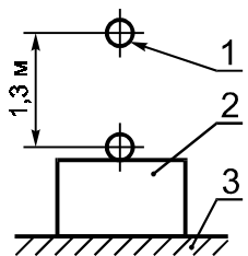
1 — стальной шарик; 2 — светильник; 3 — опорная поверхность Черт. 7а
