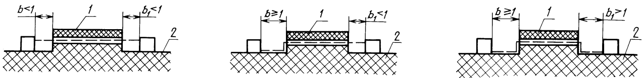
1 и 2 — детали светильника Черт. 4
