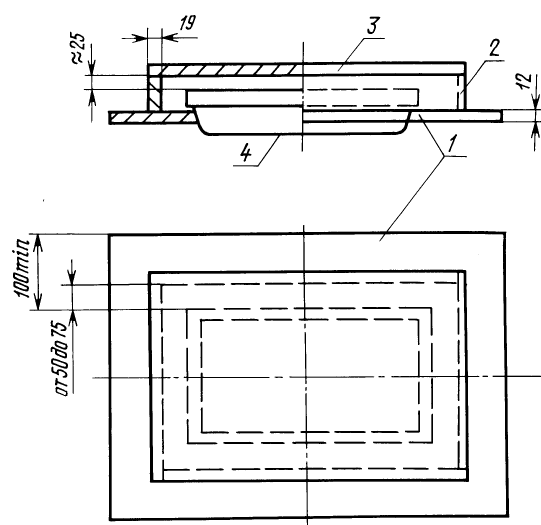
1 — основа, 2 — боковая стенка, 3 — верхняя стенка, 4 — испытываемый светильник
