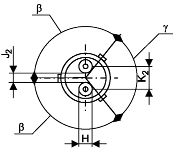
Круглые контакты
