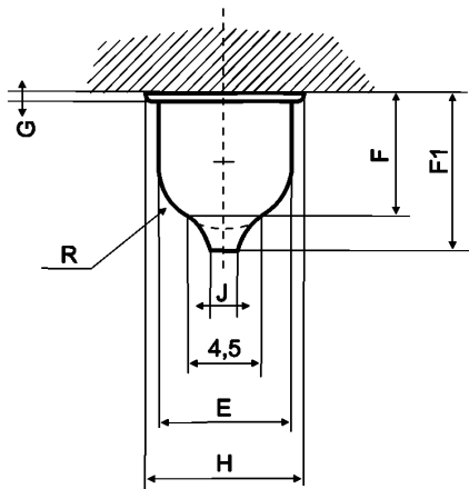
Деталь штырька
