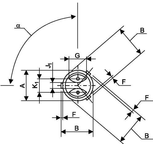
Овальные контакты
