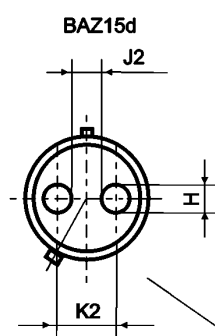
Круглые контакты
