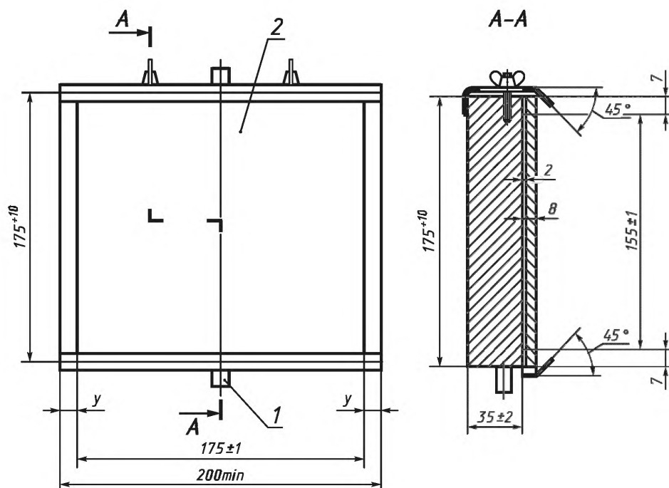
Рисунок 16 — Монтажная опора
