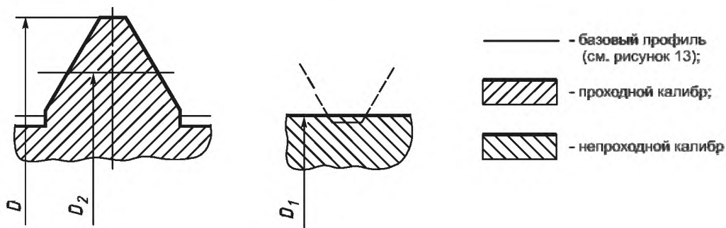
Калибры для гайки
