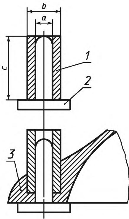
1 — втулка; 2 — вилка; 3 — основание
