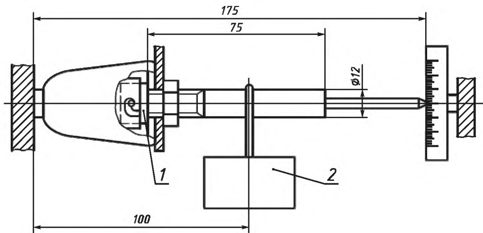
1 — испытательный цоколь; 2 — груз G
