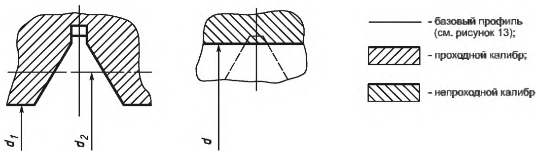
Калибры для винта
