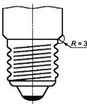
Рисунок 1 - Лампа с резьбовым цоколем
