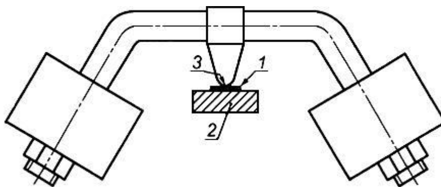
1 - образец; 2 - опора; 3 - сферический радиус 2,5 мм
