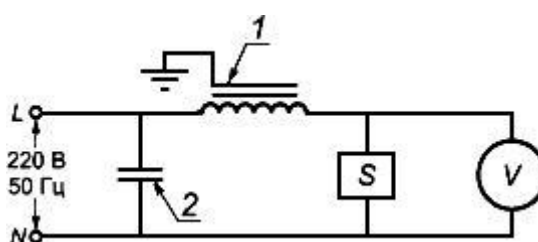
Рисунок Е.1. Схема измерения импульсов напряжения
