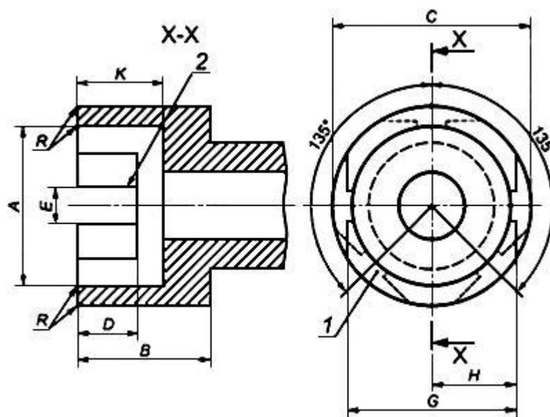
Рисунок С.2. Патрон для испытания на сопротивление крутящему моменту ламп со штифтовыми цоколями
