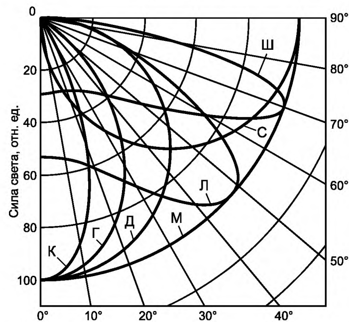
Рисунок В.1 – Типы меридиональных КСС светильников
