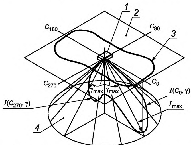
Рисунок Г.1 – Определение условной экваториальной КСС светильника
