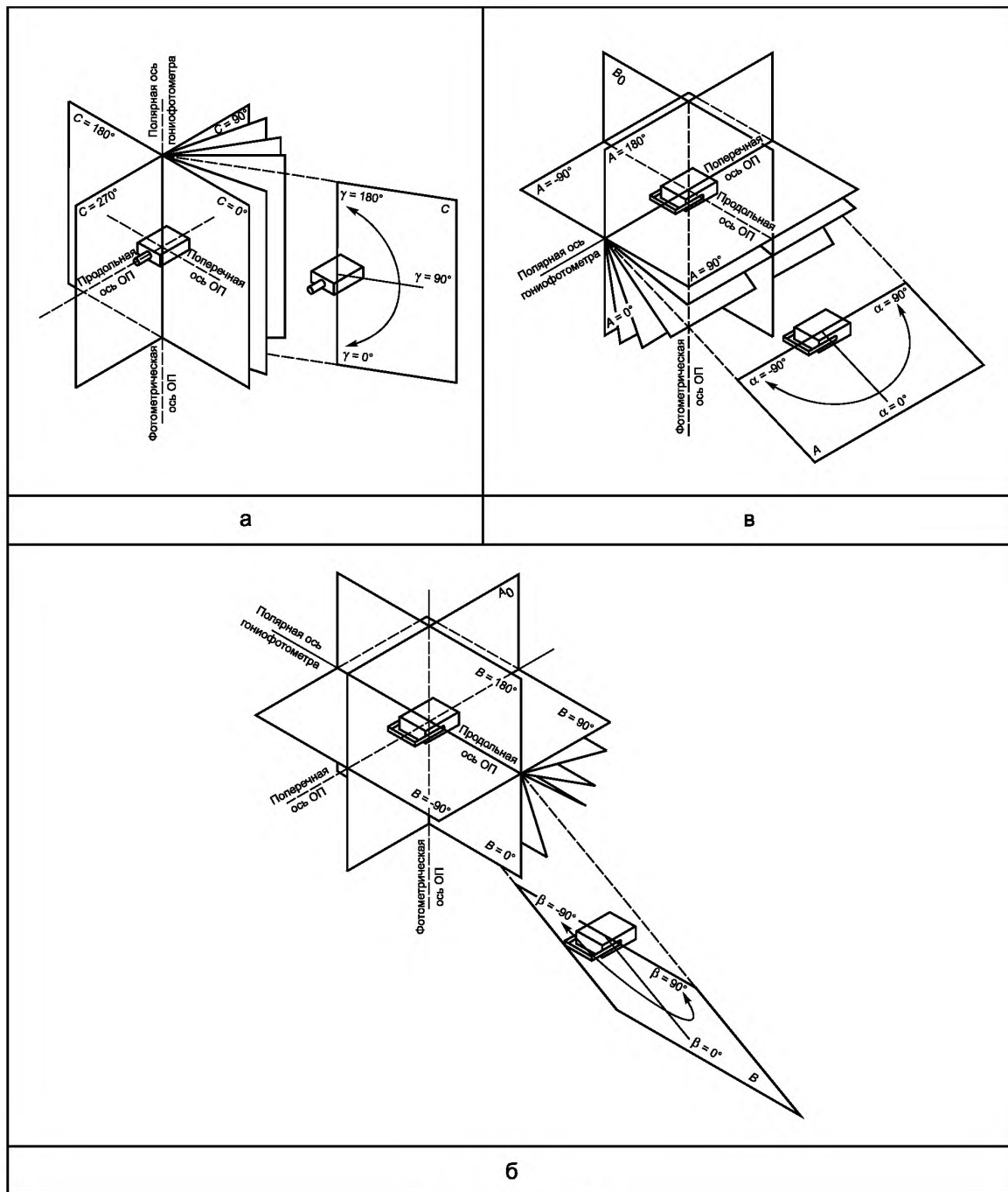
а – C - \gamma ; б – B - \beta ; в – A - \alpha
