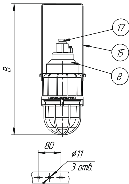
С1: на скобе
