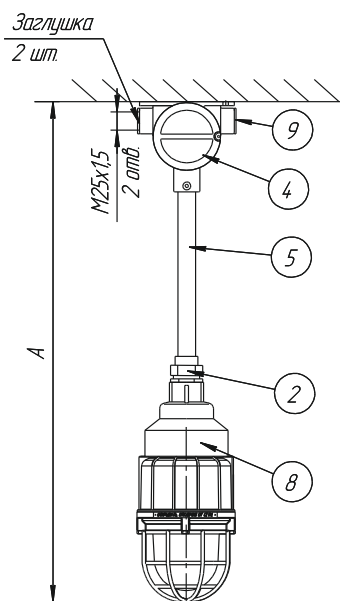
В: подвесное крепление
