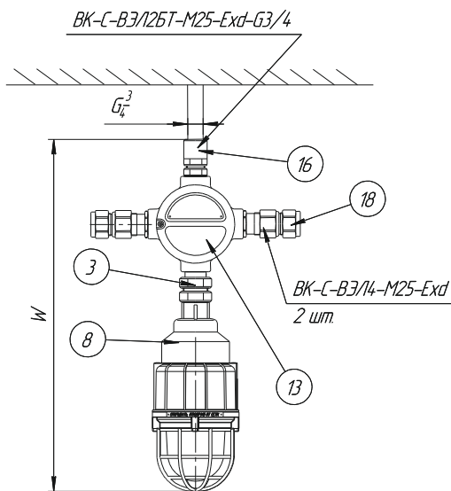
Т2: на трубе с коробкой
