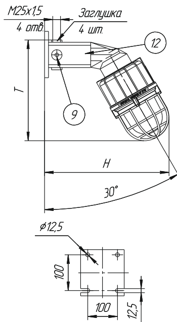
Н: настенное крепление
