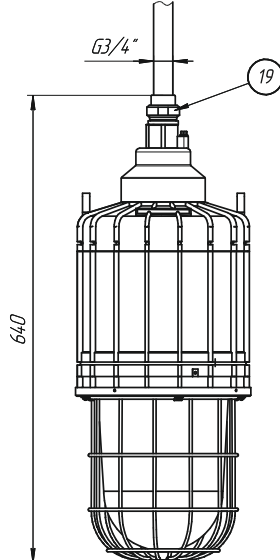
Т1: на трубе
