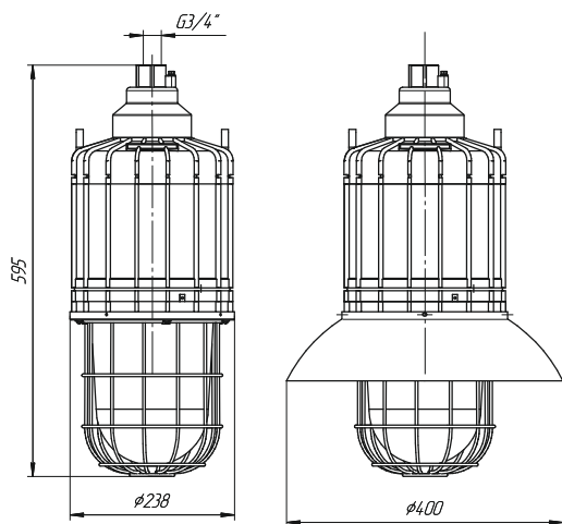
Общие размеры
