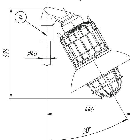
О: на опоре
