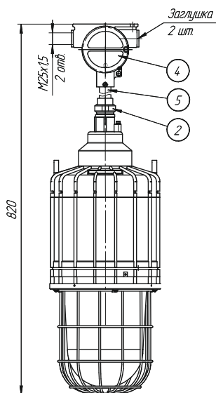
В: подвесное крепление
