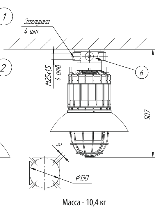
П: потолочное крепление
