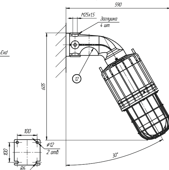
Н: настенное крепление 30°
