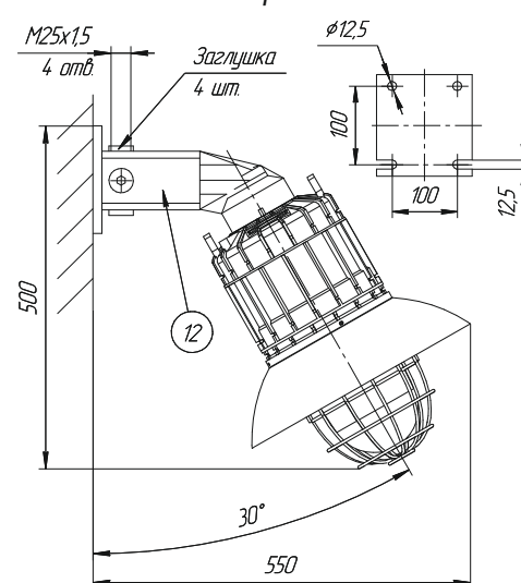
Н: настенное крепление 30°
