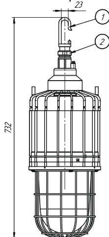
К: на крюке
