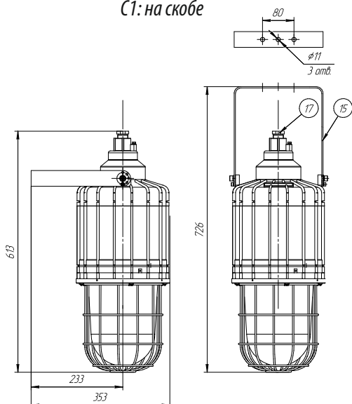
С1: на скобе
