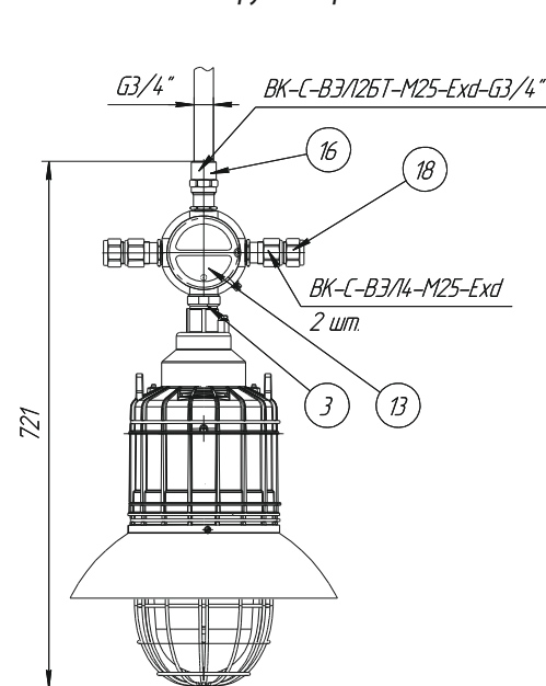
Т2: на трубе с коробкой
