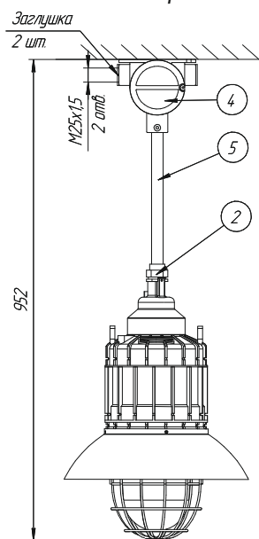
В: подвесное крепление
