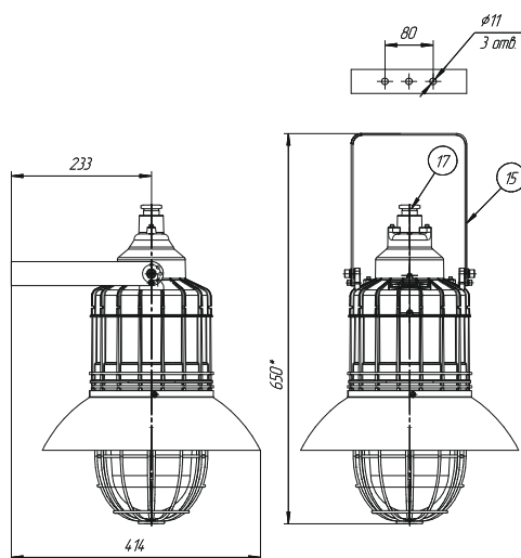
С1: на скобе
