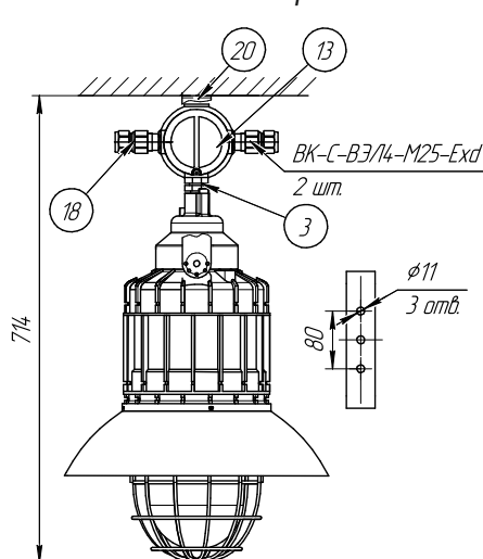
С2: на скобе с коробкой
