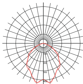
ВЭЛАН31-СД.Л.60-УХЛ1
