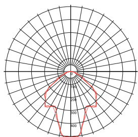
ВЭЛАН31-СД.Л.10-УХЛ1
