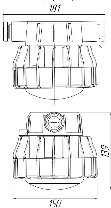
Общие размеры
