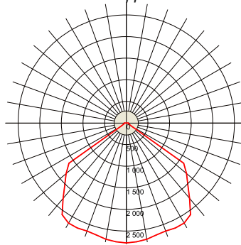
ВЭЛАН38-СД.Л.100-КО
