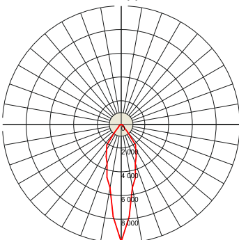
ВЭЛАН38-СД.Л.70-У
