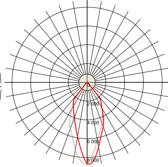
ВЭЛАН38-СД.Л.80-У
