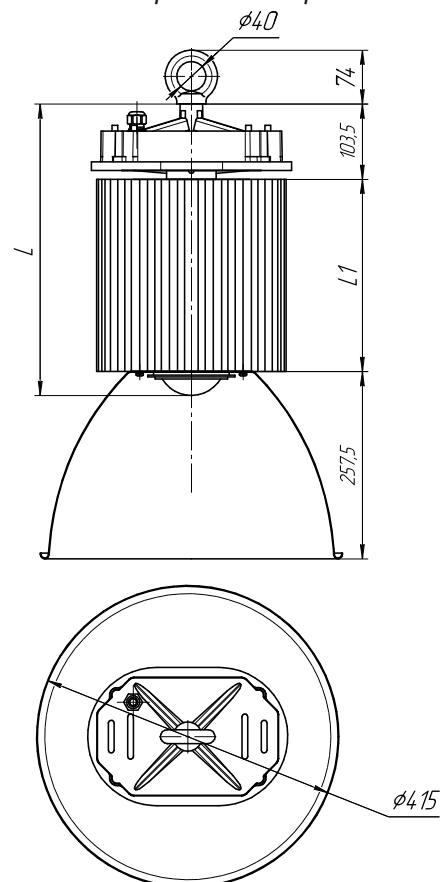
Узконаправленный отражатель
