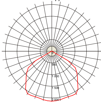
ВЭЛАН38-СД.Л.70-КО
