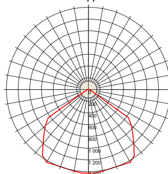
ВЭЛАН38-СД.Л.50-КО
