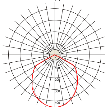
ВЭЛАН38-СД.Л.80-КО
