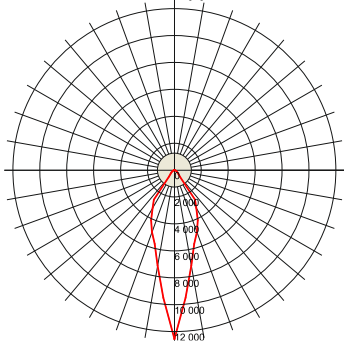
ВЭЛАН38-СД.Л.100-У
