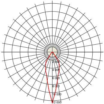
ВЭЛАН38-СД.Л.150-У
