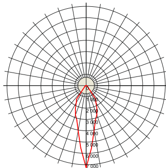
ВЭЛАН38-СД.Л.50-У
