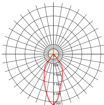
ВЭЛАН38-СД.Л.30-У
