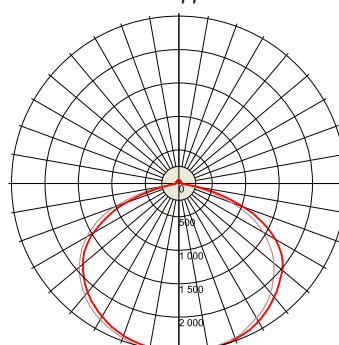
ВЭЛАН38-СД.Л.90-КО
