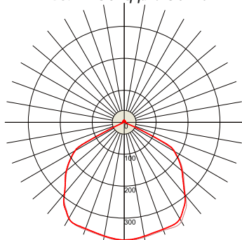
ВЭЛАН38-СД.Л.150-КО
