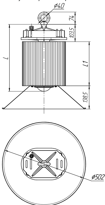
Куполообразный отражатель
