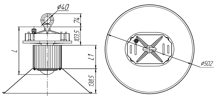
Куполообразный отражатель
