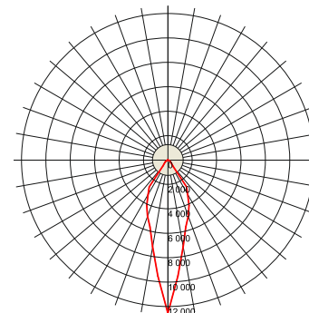
ВЭЛАН38-СД.Л.200-У
