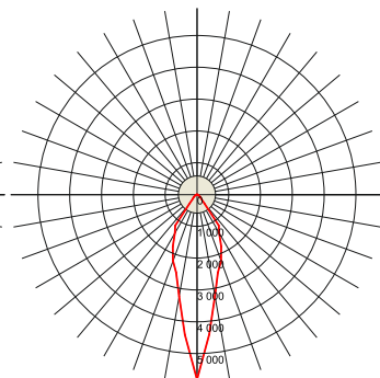
ВЭЛАН38-СД.Л.40-У
