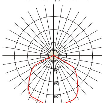
ВЭЛАН38-СД.Л.200-КО
