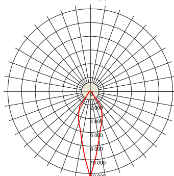
ВЭЛАН38-СД.Л.90-У
