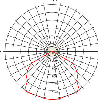
ВЭЛАН38-СД.Л.60-КО
