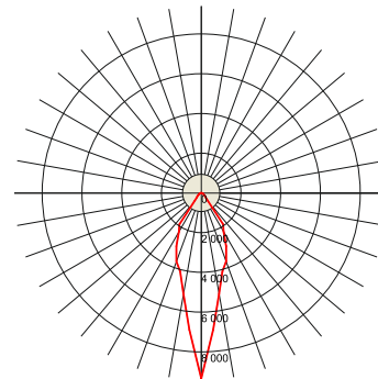
ВЭЛАН38-СД.Л.60-У
