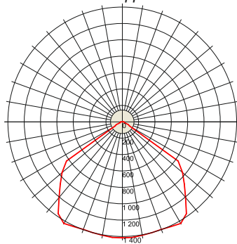
ВЭЛАН38-СД.Л.40-КО
